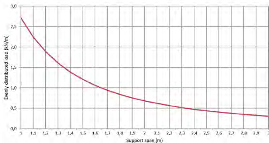
Permissible load KP 60/100 d=0,8mm (kN/m)
