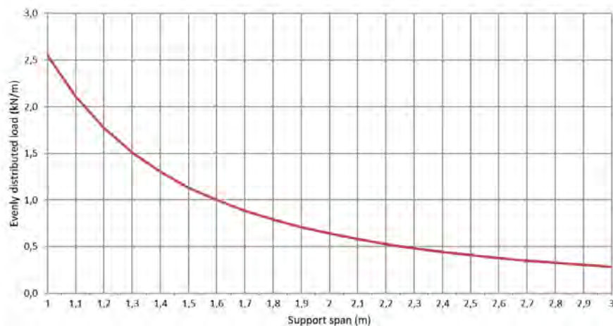
Permissible load KP 40/400 d=0,8mm (kN/m)
