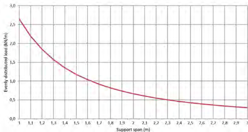
Permissible load KP 60/300 d=0,8mm (kN/m)
