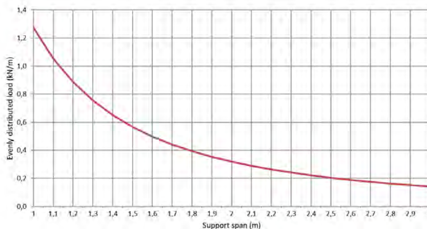
Permissible load KP 40/100 d=0,6mm (kN/m)
