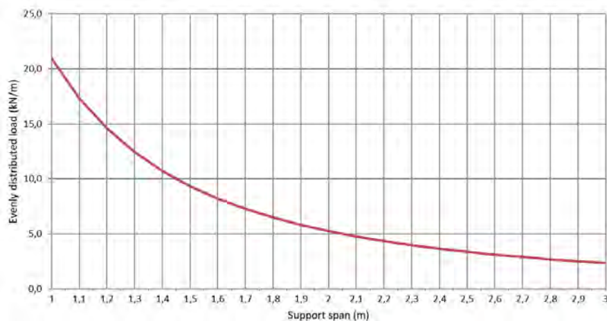
Permissible load KP 100/200 d=1,5mm (kN/m)
