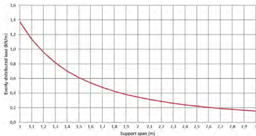
Permissible load KP 40/200 d=0,6mm (kN/m)
