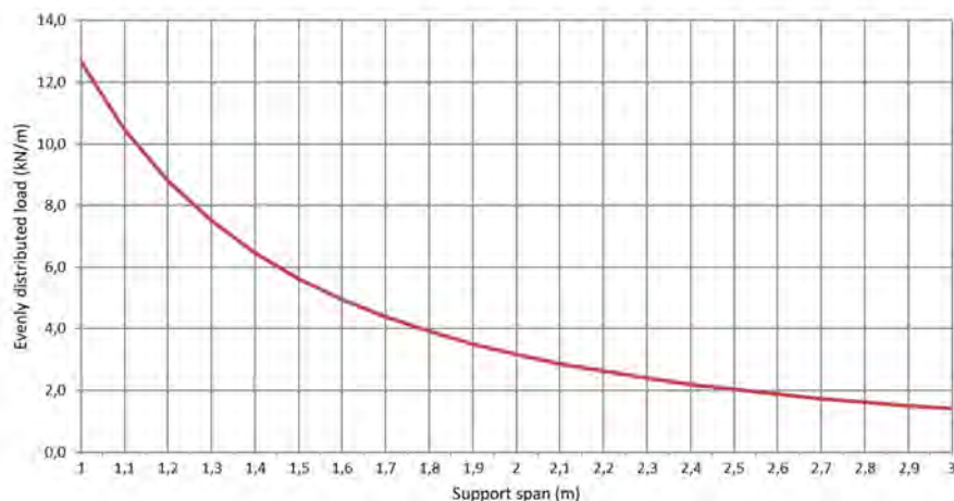
Permissible load KL 60/600 d=1,5mm (kN/m)
