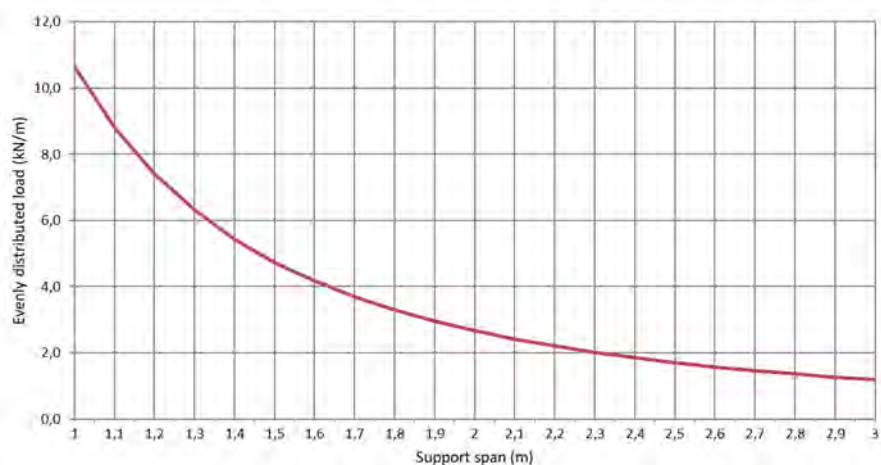
Permissible load KL 60/300 d=1,5mm (kN/m)
