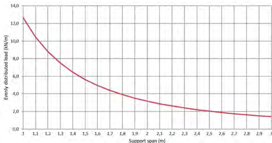
Permissible load KL 100/300 d=1,5mm (kN/m)
