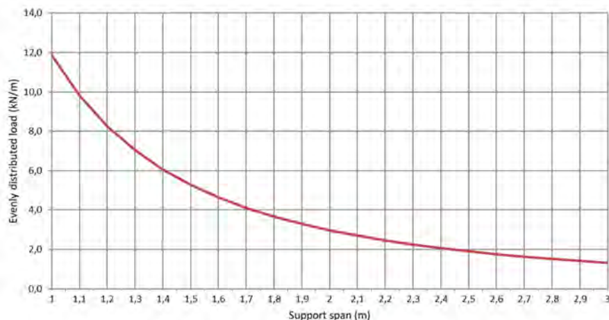
Permissible load KL 100/100 d=1,5mm (kN/m)
