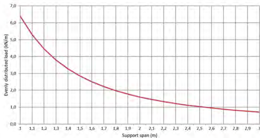
Permissible load KL 100/200 d=1,0mm (kN/m)
