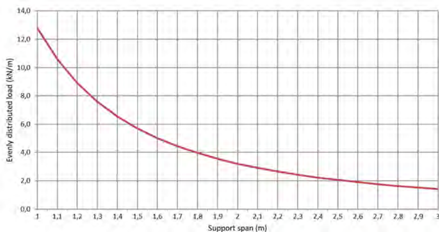
Permissible load KL 60/400 d=1,5mm (kN/m)
