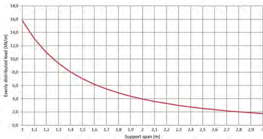
Permissible load KL 100/400 d=1,5mm (kN/m)
