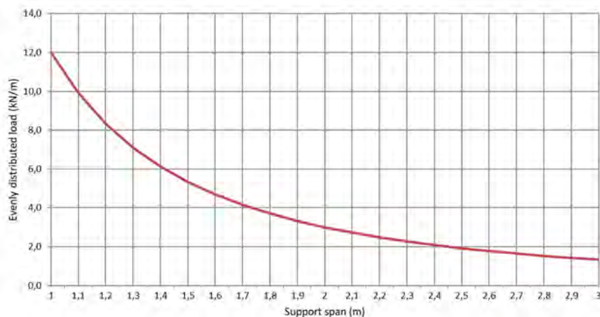
Permissible load KL 100/200 d=1,5mm (kN/m)
