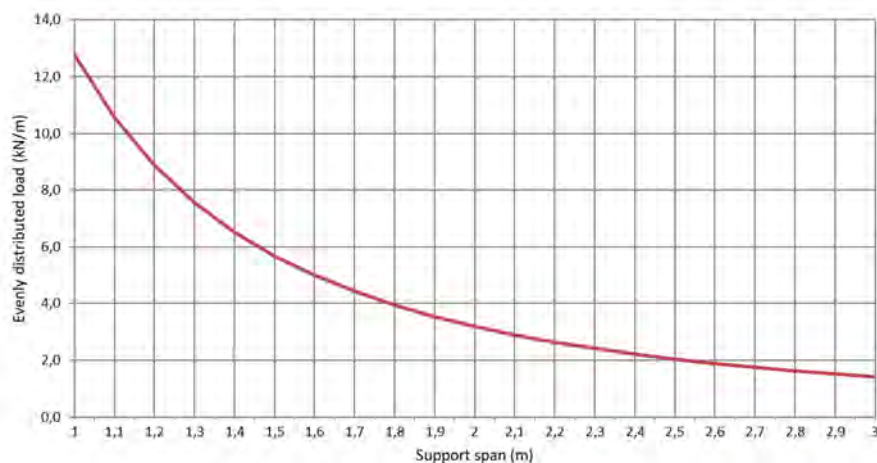
Permissible load KL 100/600 d=1,5mm (kN/m)
