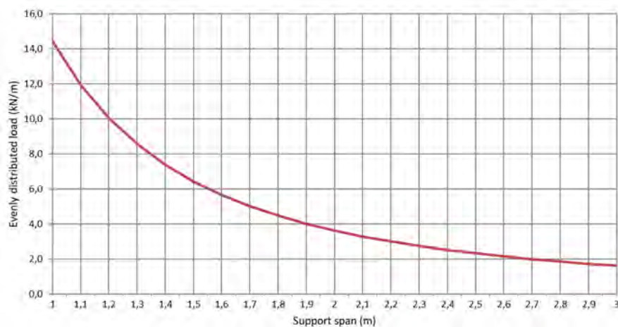
Permissible load KL 100/500 d=1,5mm (kN/m)
