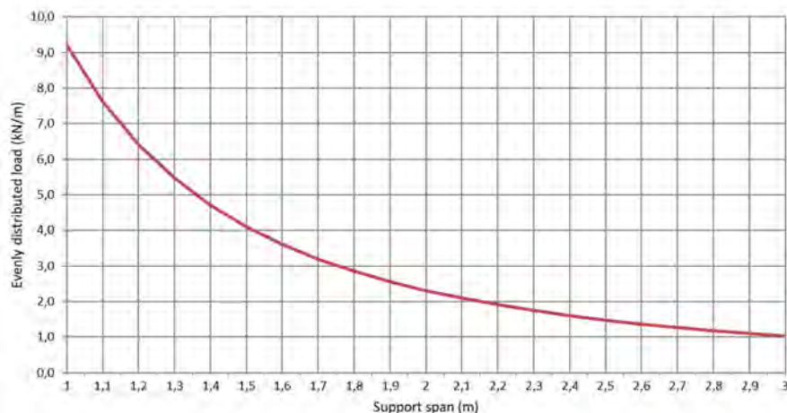
Permissible load KL 100/500 d=1,0mm (kN/m)
