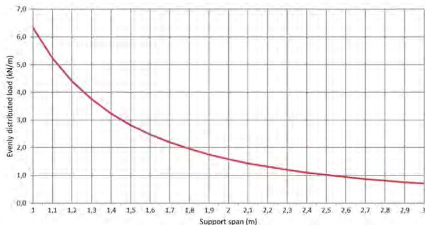
Permissible load KL 100/100 d=1,0mm (kN/m)
