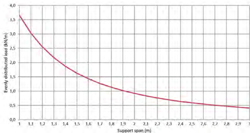
Permissible load KP 100/100 d=0,8mm (kN/m)
