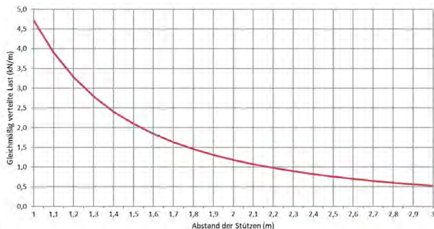
Zulässige Belastung KP 60/400 d=1,0mm (kN/m)
