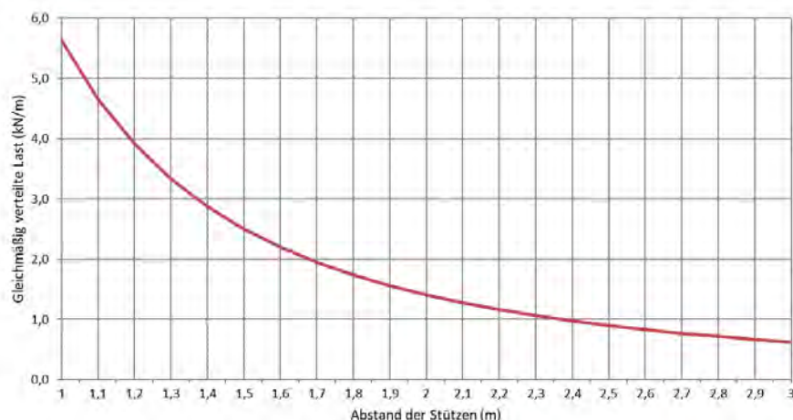
Zulässige Belastung KP 60/600 d=1,0mm (kN/m)
