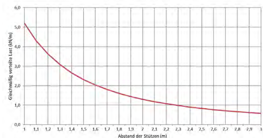
Zulässige Belastung KP 60/500 d=1,0mm (kN/m)
