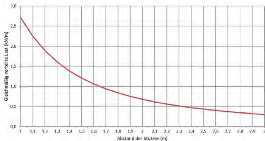
Zulässige Belastung KP 60/100 d=0,8mm (kN/m)
