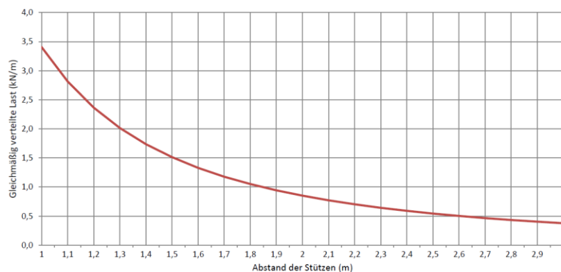
Zulässige Belastung KPK 100/100 d=0,75mm (kN/m)
