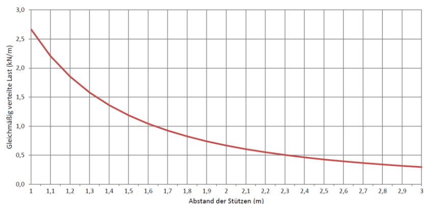
Zulässige Belastung KPK 80/100 d=0,75mm (kN/m)
