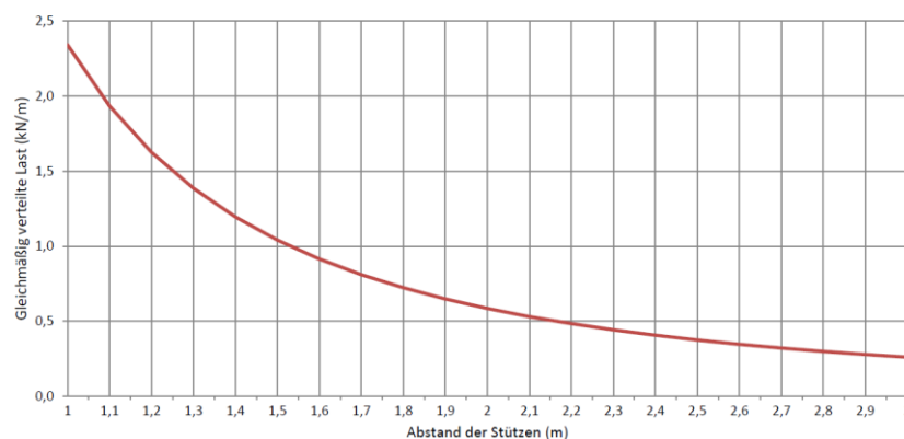
Zulässige Belastung KPK 60/100 d=0,75mm (kN/m)
