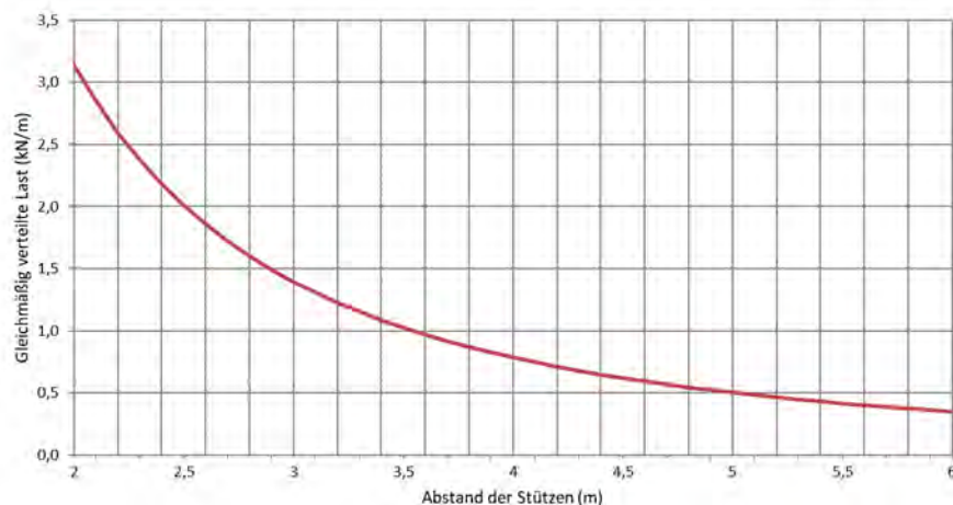
Zulässige Belastung KL HD 100/600 d=1,5mm (kN/m)
