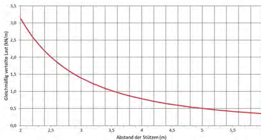
Zulässige Belastung KL HD 100/600 d=1,5mm (kN/m)
