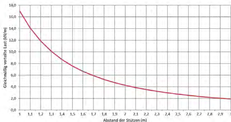
Zulässige Belastung KP 100/600 d=1,5mm (kN/m)
