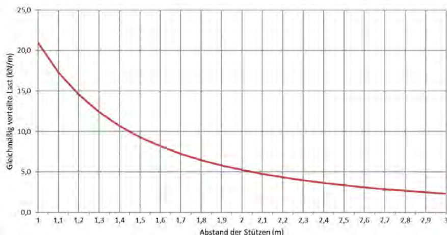
Zulässige Belastung KP 100/200 d=1,5mm (kN/m)
