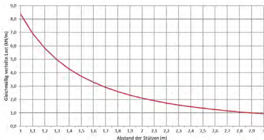
Zulässige Belastung KP 60/200 d=1,5mm (kN/m)
