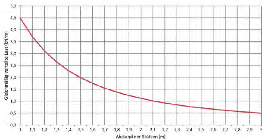
Zulässige Belastung KP 60/300 d=1,0mm (kN/m)
