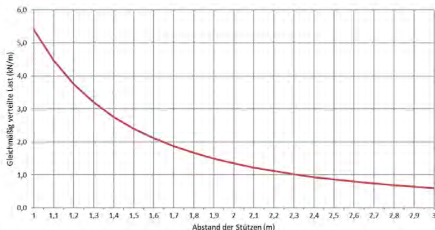
Zulässige Belastung KP 100/600 d=1,0mm (kN/m)
