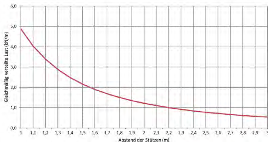
Zulässige Belastung KP 100/300 d=1,0mm (kN/m)
