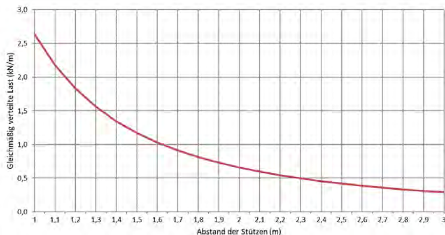
Zulässige Belastung KP 40/600 d=0,8mm (kN/m)
