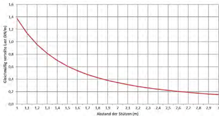
Zulässige Belastung KP 40/200 d=0,6mm (kN/m)
