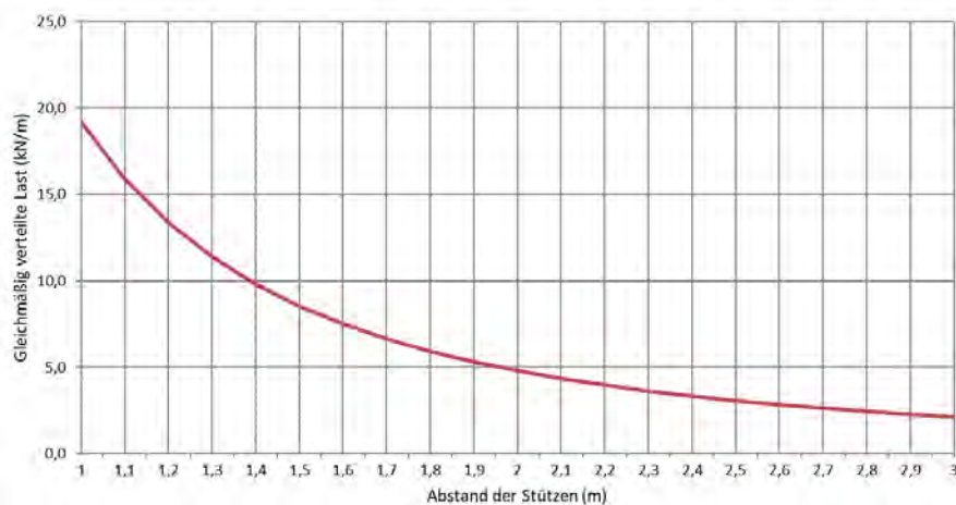
Zulässige Belastung KP 100/500 d=1,5mm (kN/m)
