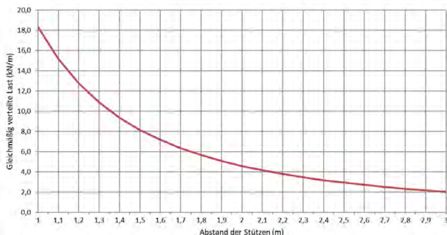
Zulässige Belastung KP 100/400 d=1,5mm (kN/m)
