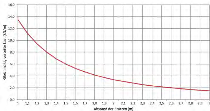
Zulässige Belastung KP 60/600 d=1,5mm (kN/m)
