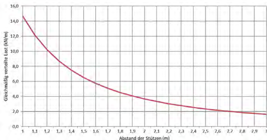
Zulässige Belastung KP 60/500 d=1,5mm (kN/m)
