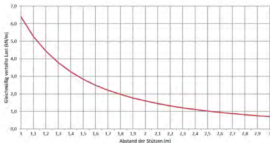
Zulässige Belastung KP 100/500 d=1,0mm (kN/m)
