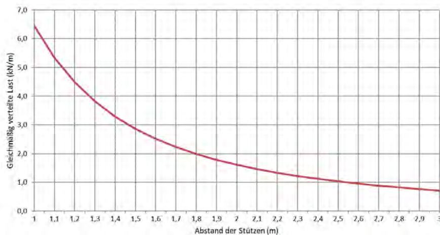
Zulässige Belastung KP 100/400 d=1,0mm (kN/m)
