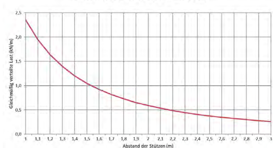
Zulässige Belastung KP 40/500 d=0,8mm (kN/m)
