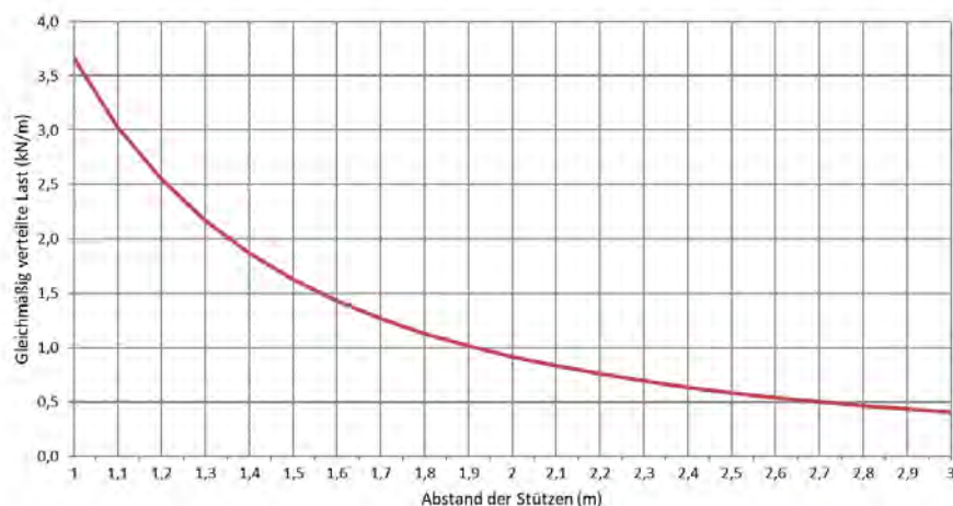
Zulässige Belastung KP 100/100 d=0,8mm (kN/m)
