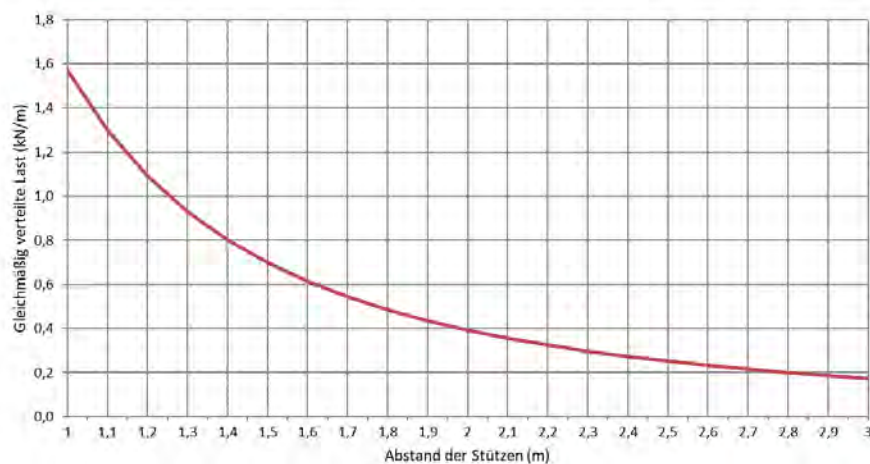
Zulässige Belastung KP 60/150 d=0,6mm (kN/m)
