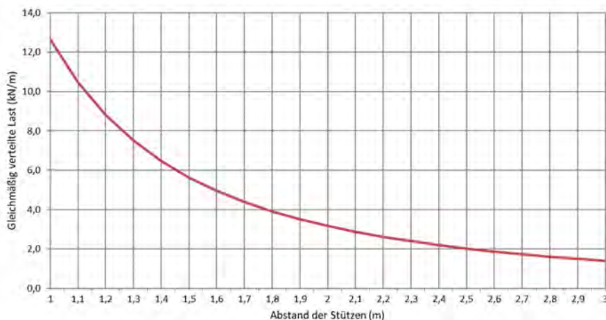
Zulässige Belastung KL 60/600 d=1,5mm (kN/m)
