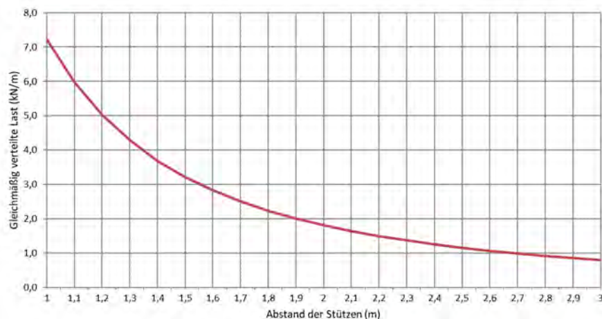
Zulässige Belastung KL 100/600 d=1,0mm (kN/m)
