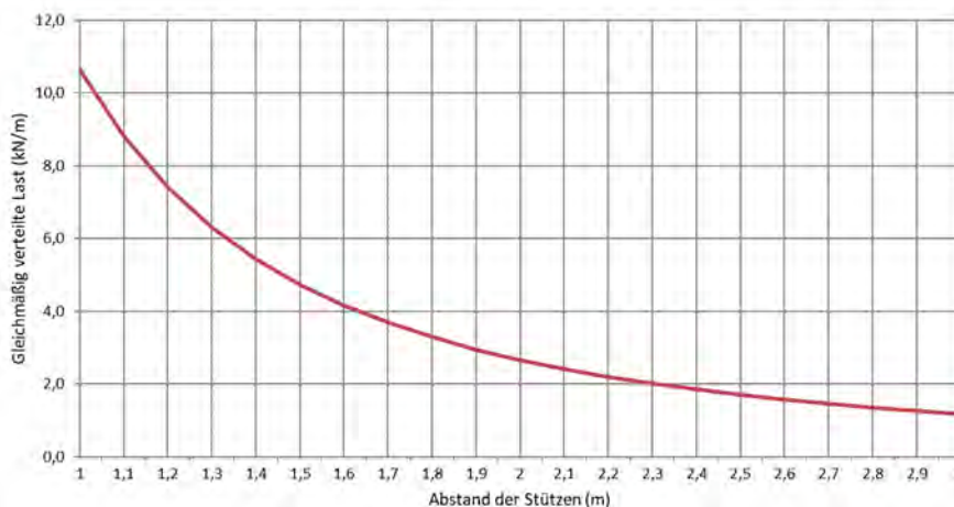
Zulässige Belastung KL 60/300 d=1,5mm (kN/m)
