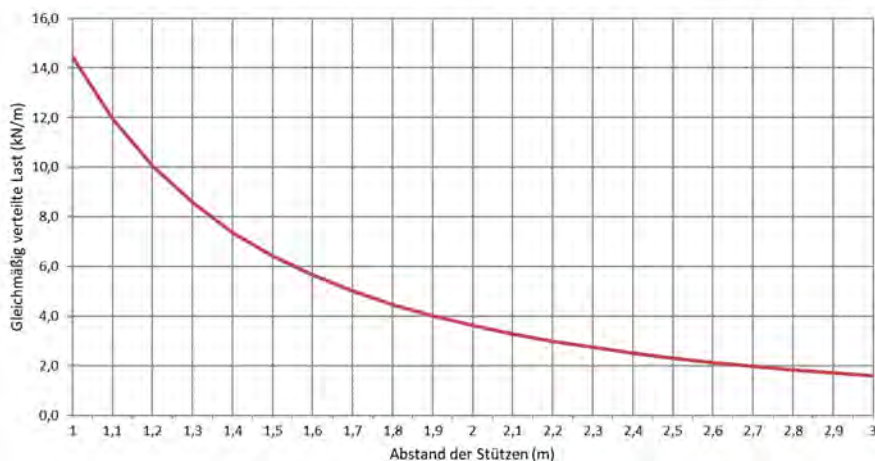
Zulässige Belastung KL 100/500 d=1,5mm (kN/m)
