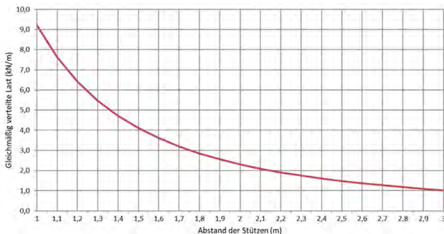
Zulässige Belastung KL 100/500 d=1,0mm (kN/m)
